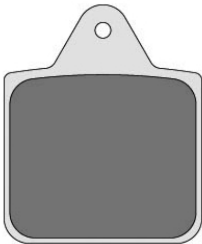
DB 2600 50,4x60,8x12,3
