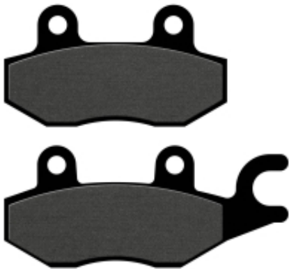
FD117 (16, 7,5mm) non replace FD145 (not vice versa) | FD117 (16, 7,5mm) puede sustituir FD145 (no al revés)
